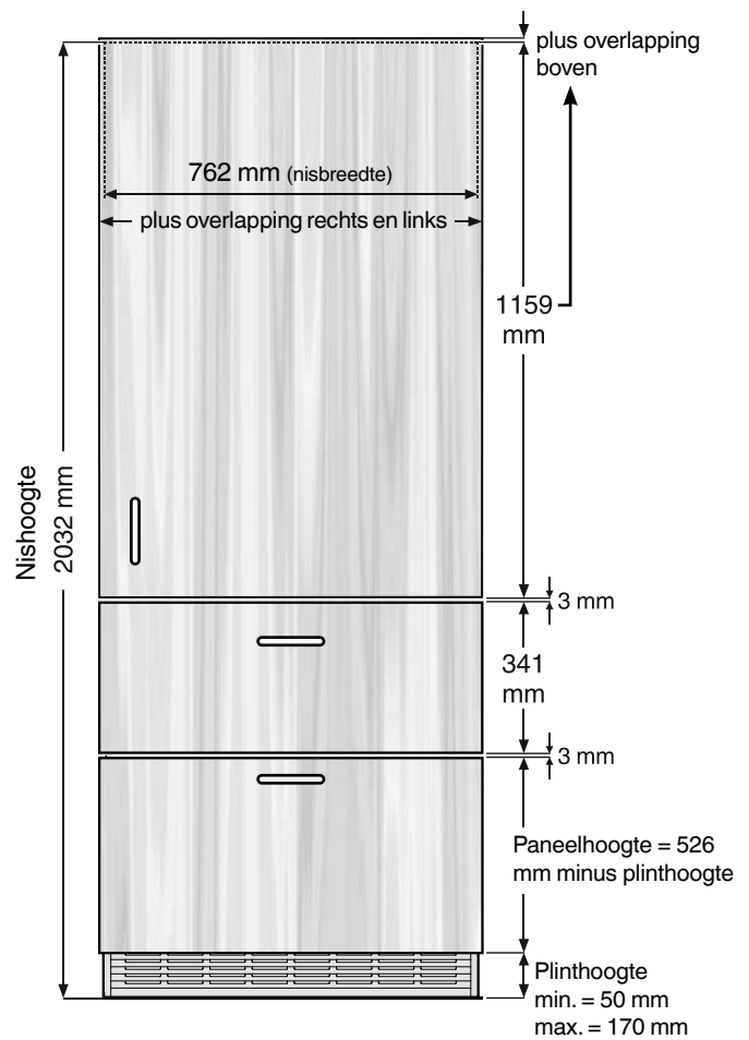
Buitenliggend deurpaneel
