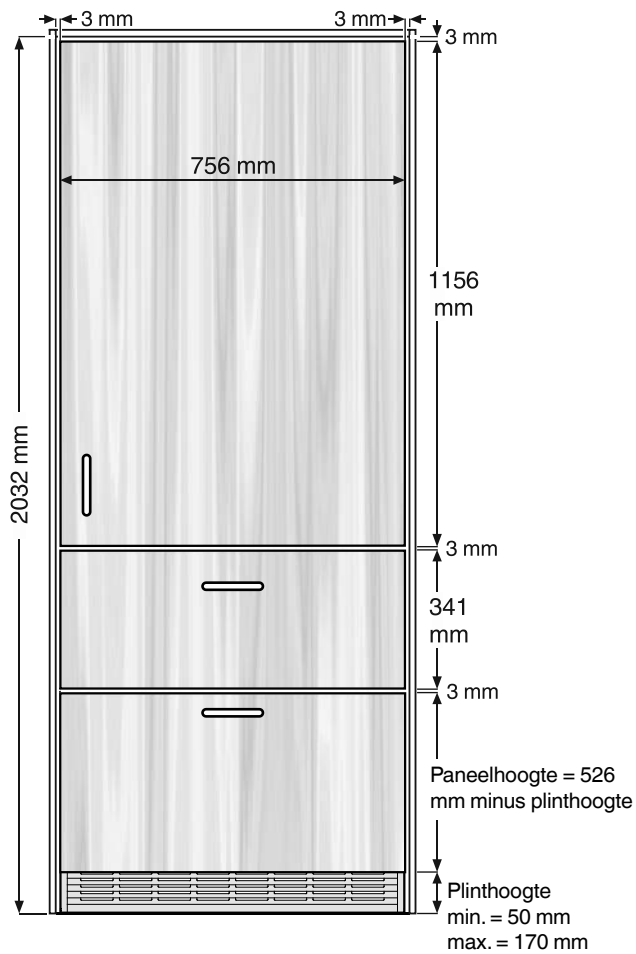
Binnenliggend deurpaneel
