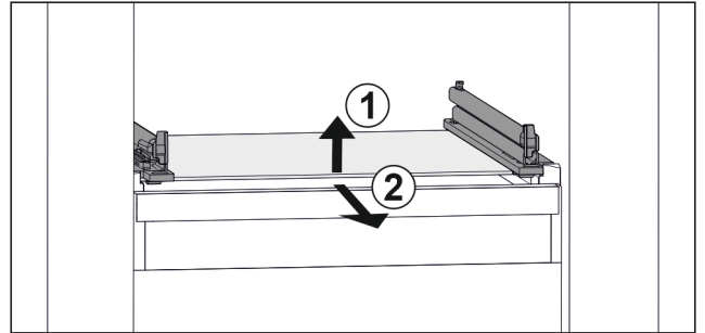
Fig. 72 Lasihyllyn esimerkinomainen kuvaus
