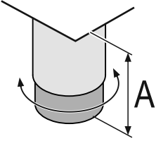
Fig. 12 Το ρυθμιζόμενο πόδι μπορεί να ρυθμιστεί από A = 115 \text{ mm} (4 1/2 in) έως 175 \text{ mm} (6 7/8 in).
