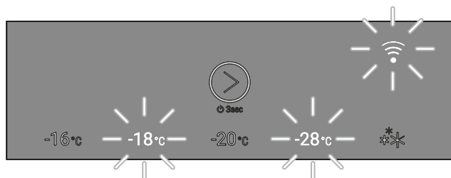
Fig. 46 Ekrani në gabimin e WLAN
