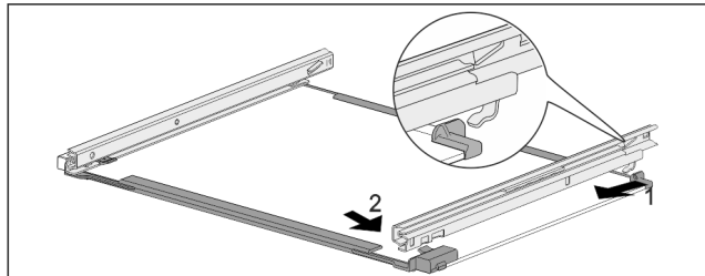
Fig. 113 Steklена plošča z vodili
