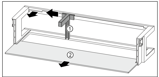
Fig. 93 Vratna polica z držalom za steklenice in odlagalno polico
