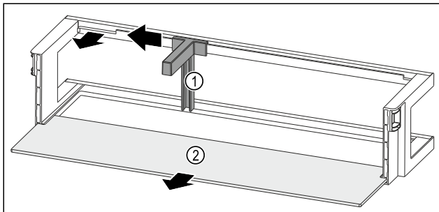
Fig. 90 Türabsteller mit Flaschenhalter und Abstellfläche
