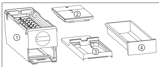
Fig. 80 Bestandteile des EasyTwist-Ice
