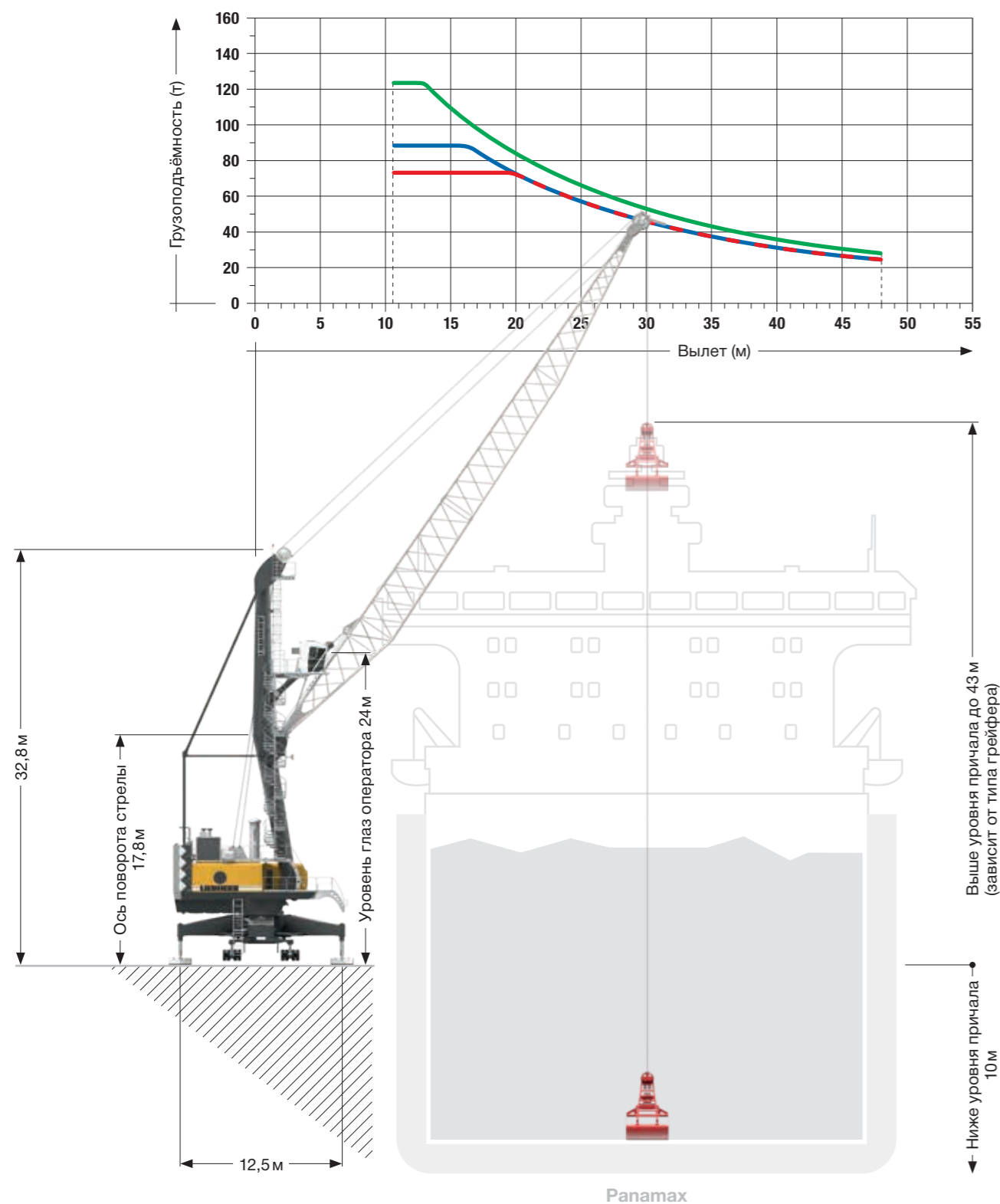
Диаграмма грузоподъёмности
