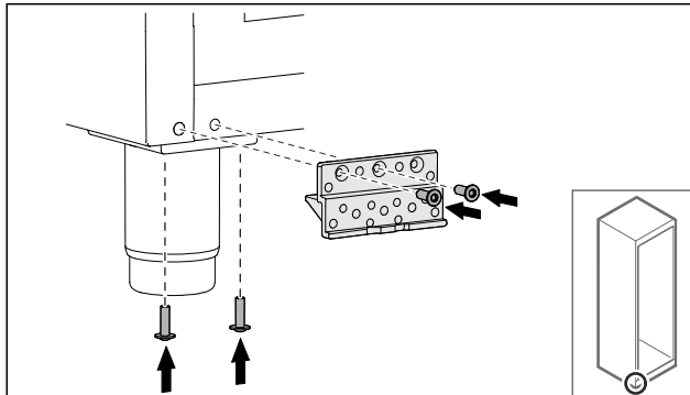
Fig. 37 ► Skru på lagerbukk. ▷ Lagerbukken er flyttet.
