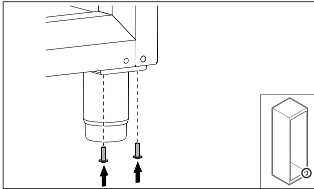
Fig. 36 ► Skru på skruer.
