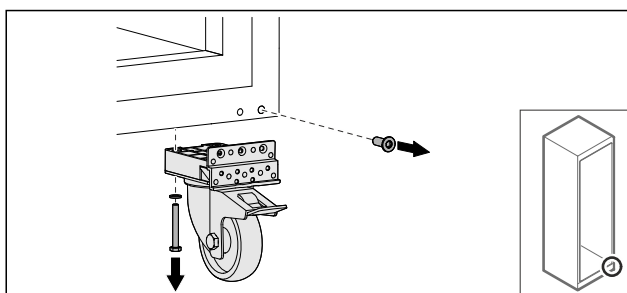
Fig. 38 ► Skru av ruller.
