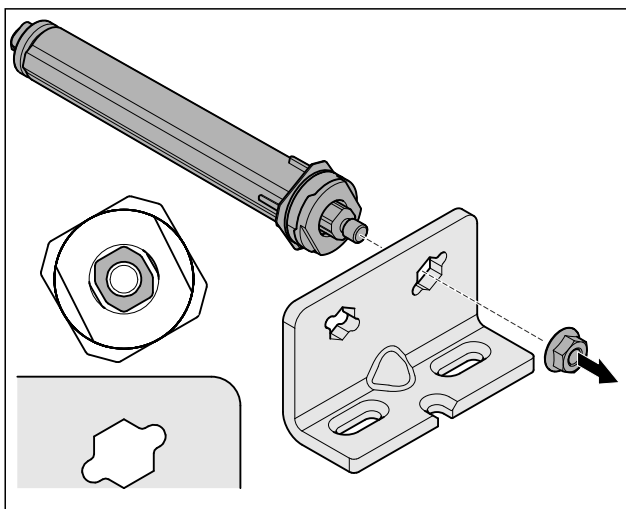
Fig. 24 Høyreanslag
