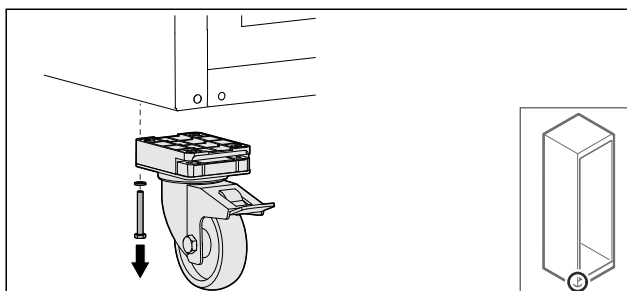
Fig. 39 ► Skru av ruller med lagerbukk.
