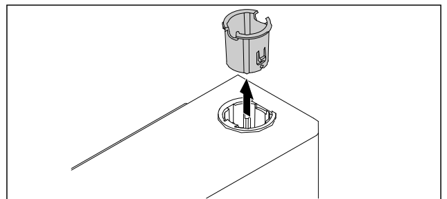
Fig. 43 ► Trekk ut hengselbøssingen på motsatt side.
