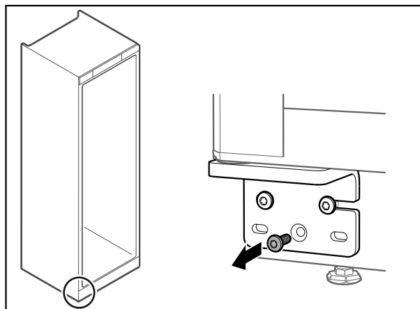
Fig. 73 Congélateur
