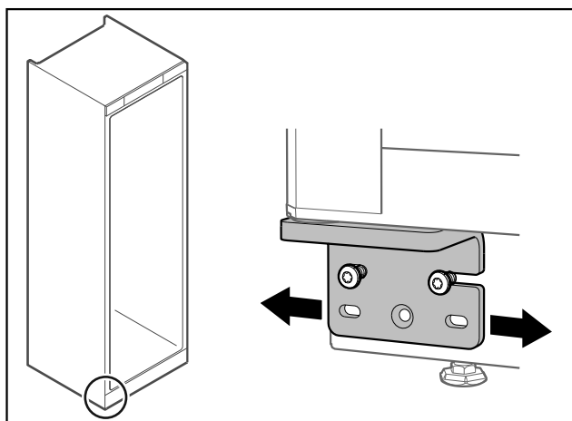
Fig. 74 Congélateur
