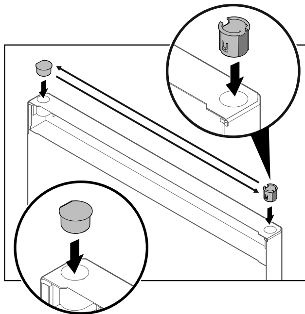
Fig. 43 Porte de la partie congélateur
