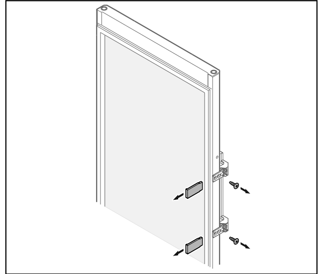
Fig. 38 Porte vitrée*
