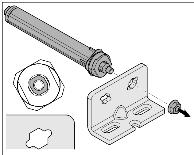
Fig. 23 Battuta a destra
