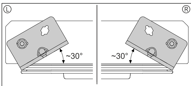
Fig. 43 Porta vista da sotto
