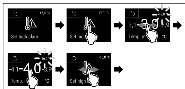
Fig. 174 Esempio di regolazione del limite inferiore di temperatura, sulla base della temperatura impostata dell'apparecchio di -20 °C.
