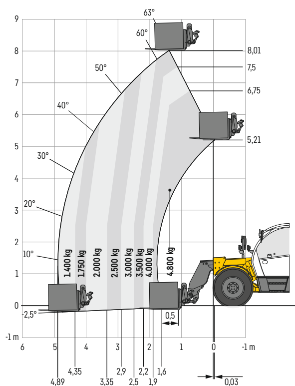
T 48-8s mit Pendelachssperre
