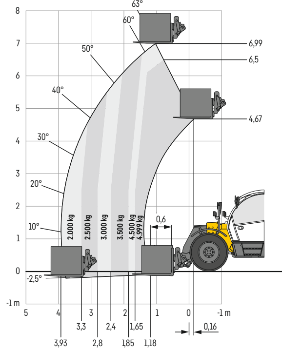
T 60-9s mit Pendelachssperre
