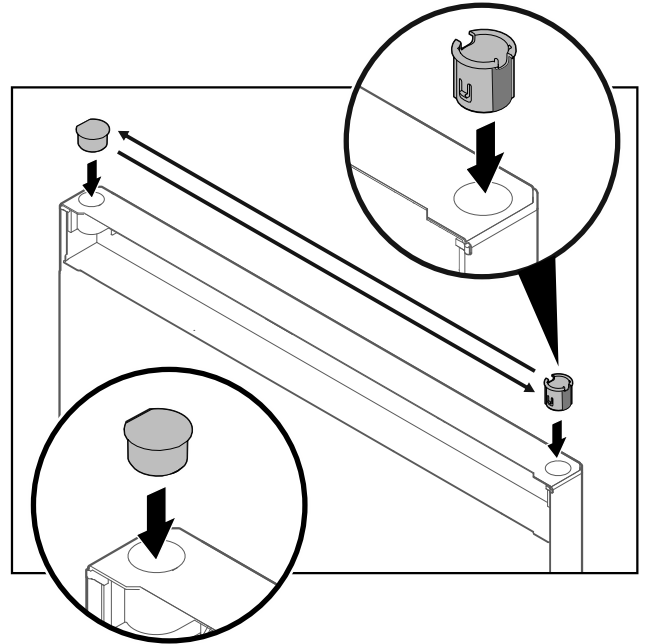
Fig. 29 Πόρτα τμήματος συντήρησης
