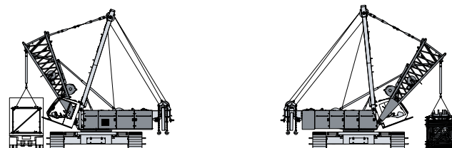
Déchargement et assemblage de la flèche
