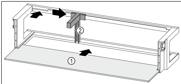
Фиг. 53 Полица на вратата со склад
