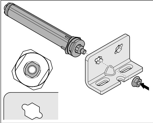
Fig. 32 左止挡
