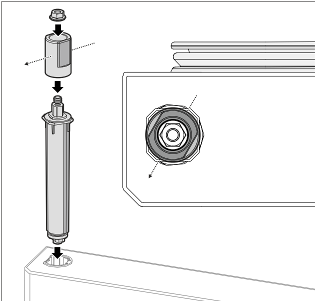
Fig. 57 左止挡
