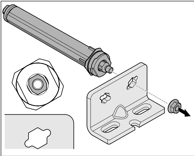
Fig. 30 右止挡
