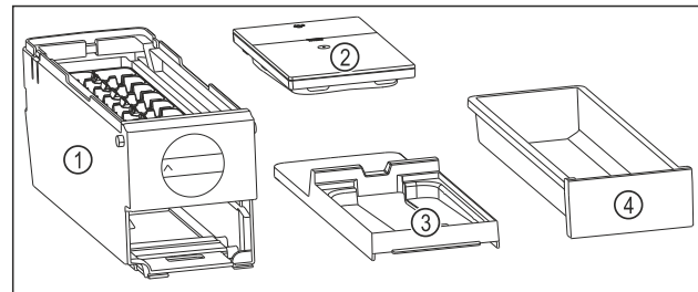
Fig. 143 Beståndsdelar i EasyTwist-Ice
