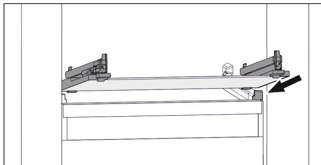
Fig. 124 Exempel på glashylla
