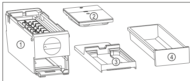
Fig. 143 Dele af EasyTwist-Ice
