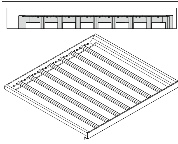
Fig. 90 Placering af lister til maks. antal flasker.
