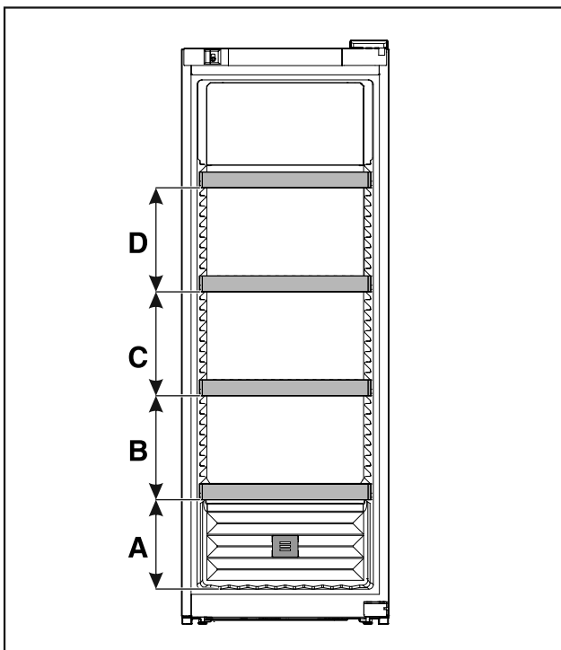
Fig. 12 Abstände Auflageroste
