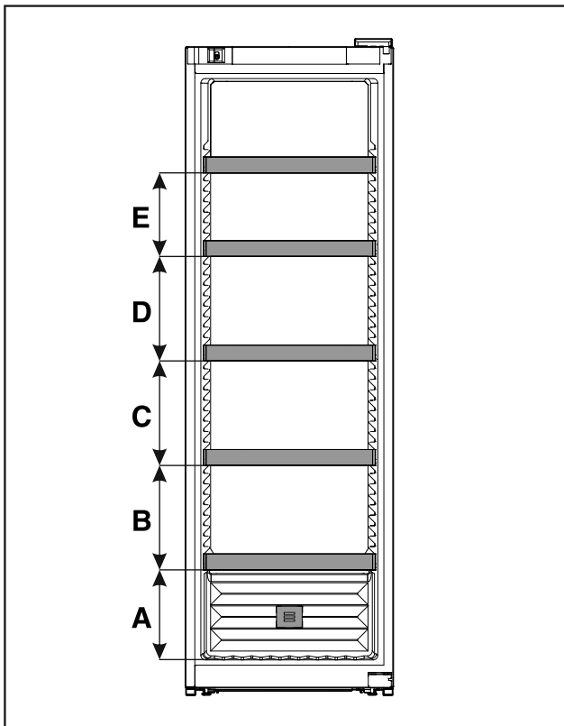
Fig. 14 Abstände Auflageroste
