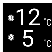
Fig. 14 Stavová obrazovka*
