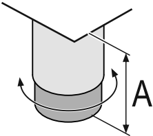
Fig. 10 Ніжка регулюється в діапазоні від A = 115 мм (4 1/2 in) до 175 мм (6 7/8 in).
