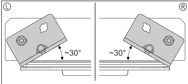
Fig. 47 从底部看门
