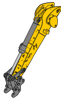
Scherenstiel
