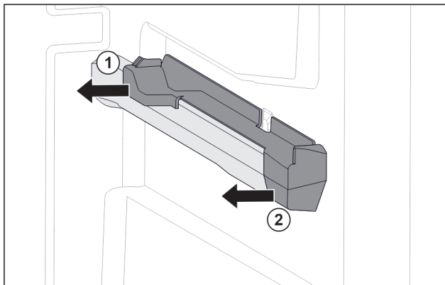
Fig. 77 Uzspraužamā daļa uz labās tvertnes ribas
