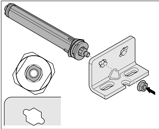
Fig. 26 Lavý doraz
