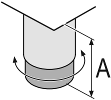
Fig. 12 Säädettävä jalka on säädettävissä A = 115 \text{ mm (4 1/2 tuumaa)} - 175 \text{ mm (6 7/8 tuumaa)} .
