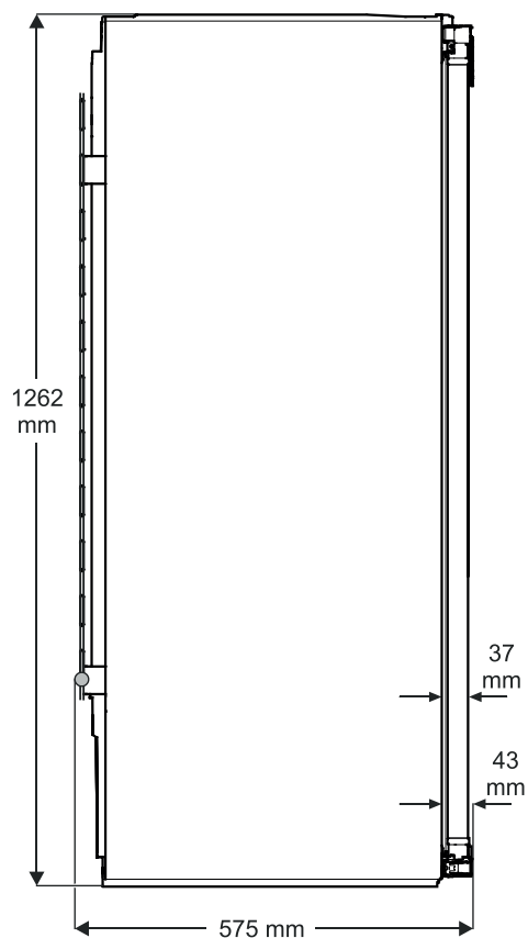
Vista laterale
