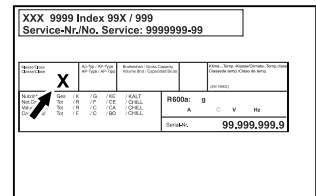
Fig. 4 Datu plāksnīte
