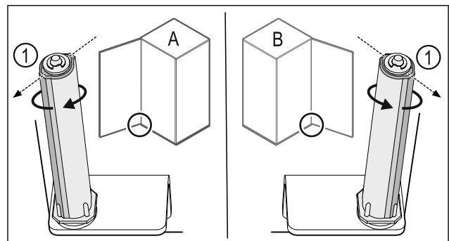
Fig. 55 Μεντεσέδες αριστερά (A) / Μεντεσέδες δεξιά (B)
