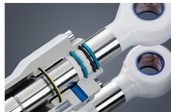
液压油缸
